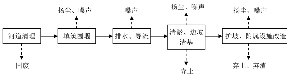
图 5-1 本项目施工工艺流程及产污节点图
